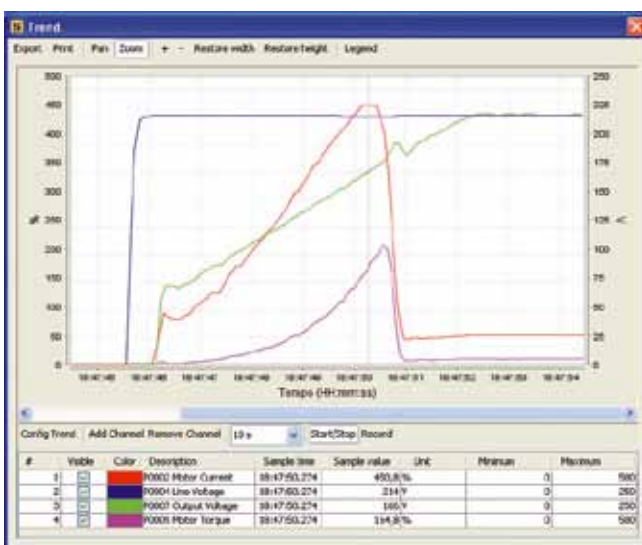
Función trace.
